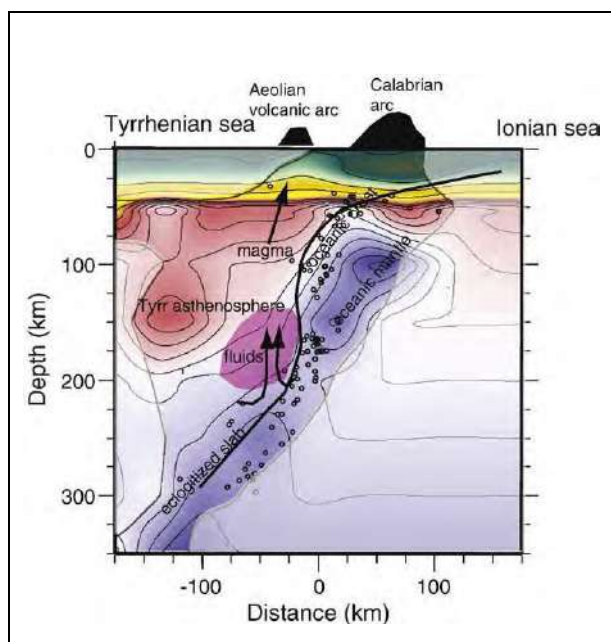
Fig. 1 - Sezione del mantello superiore dallo Ionio al Tirreno, con l'evidenza del piano di subduzione, marcato sia dalla sismicità che dall'anomalia positiva di velocità (da Chiarabba et al., 2008).
