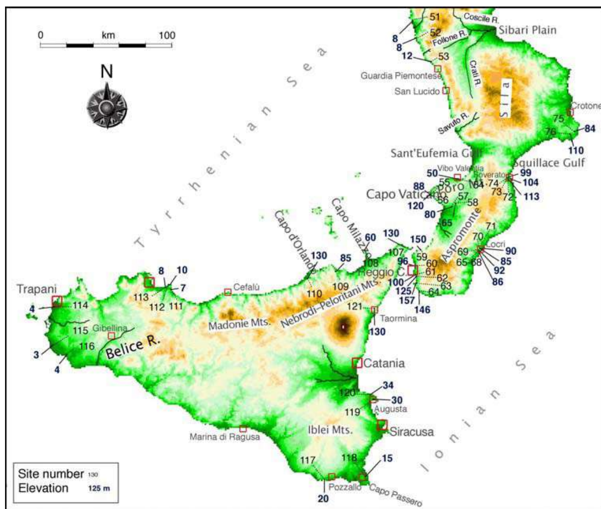
Fig. 3 - Quota attuale in metri (numeri in grassetto) della linea di riva del Tirreniano (125.000 anni) in Calabria e Sicilia. Questo importante marker del paesaggio è utilizzato per comprendere in dettaglio l'andamento del sollevamento a cui è ancora oggi sottoposta l'intera regione. Il sollevamento è massimo nella zona dello Stretto di Messina, raggiunge valori di 150 metri nell'area di Scilla, e tende ad azzerarsi procedendo verso il confine calabrolucano, verso l'area iblea e verso l'estremità occidentale della Sicilia (Bordoni e Valensise, 1998).
